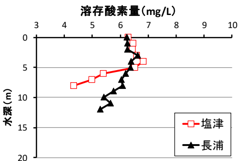
図 2. 各養殖場における水温・塩分・溶存酸素量の鉛直分布【8月1日観測】
