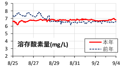
図2. 水深10mの水温・溶存酸素量の推移 (8月25日～9月4日の観測ブイの結果)
