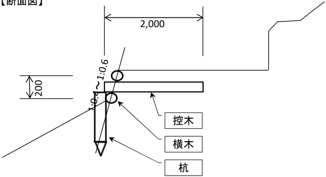
【断面図】
