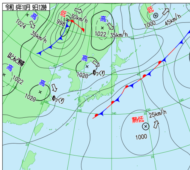
9日 12時 実況天気図
