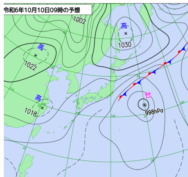
10日 9時 予想天気図
