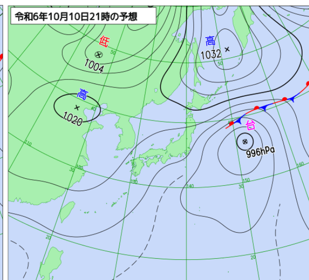
10日 21時 予想天気図
