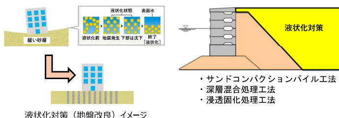
液状化対策（地盤改良）イメージ
