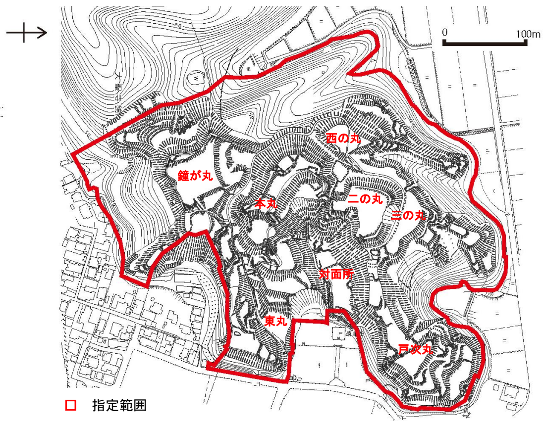
大聖寺城跡 配置図
