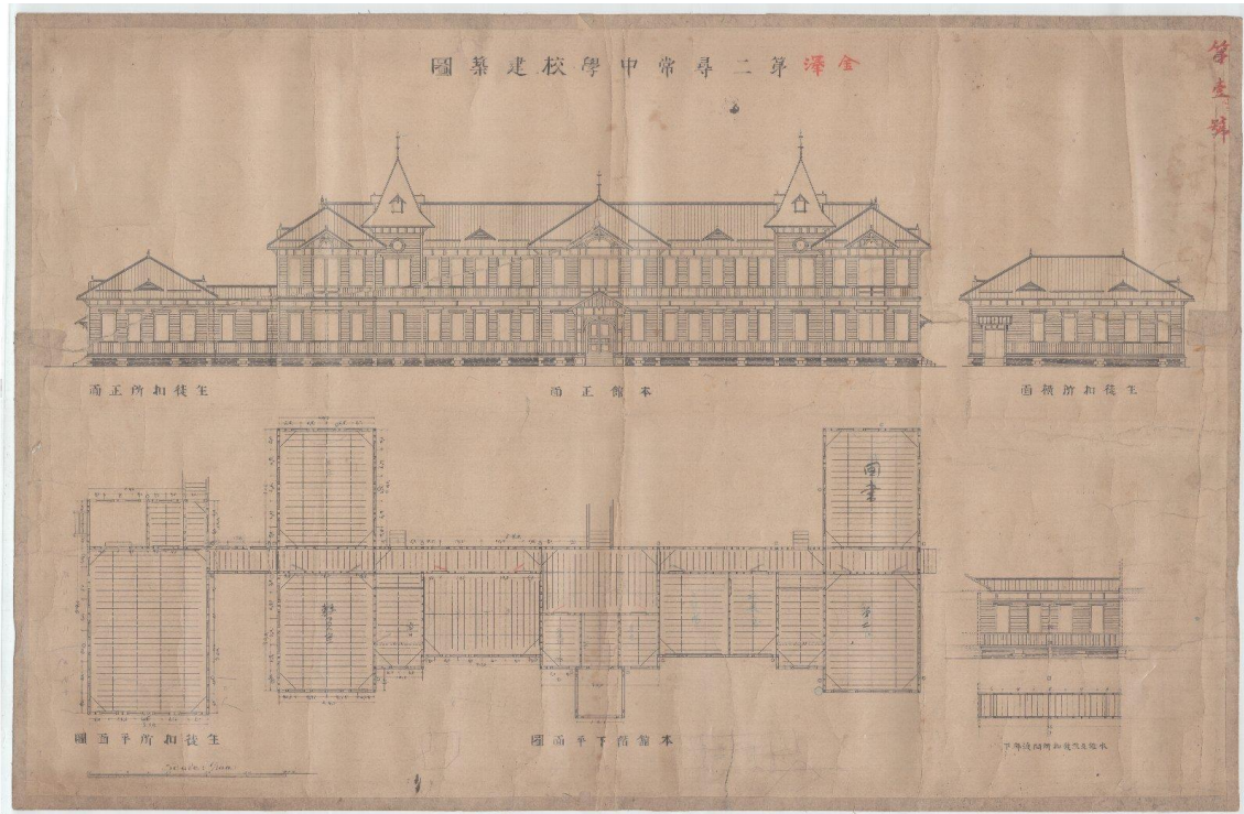
金沢第二尋常中學校建築圖
