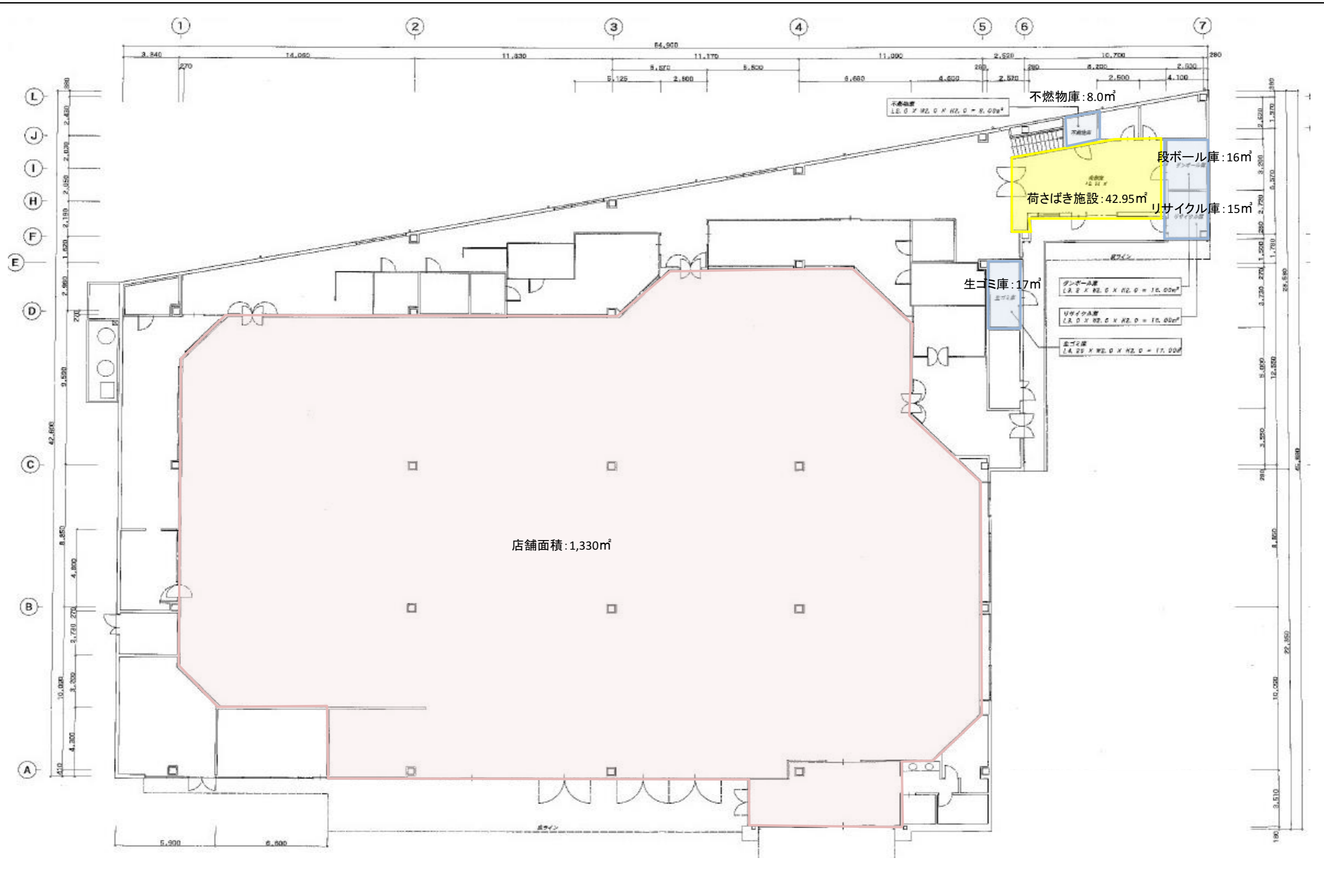
図5-1 1階平面図(変更前) 1/200
