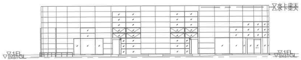
西側立面図
