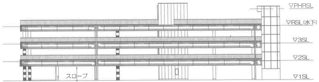
東側立面図
