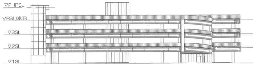
西側立面図
