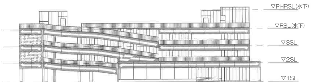
南側立面図
