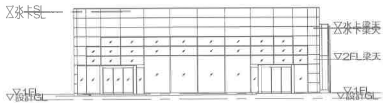
南側立面図
