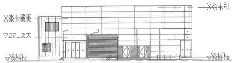
北側立面図
