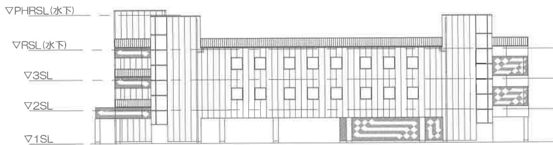
北側立面図
