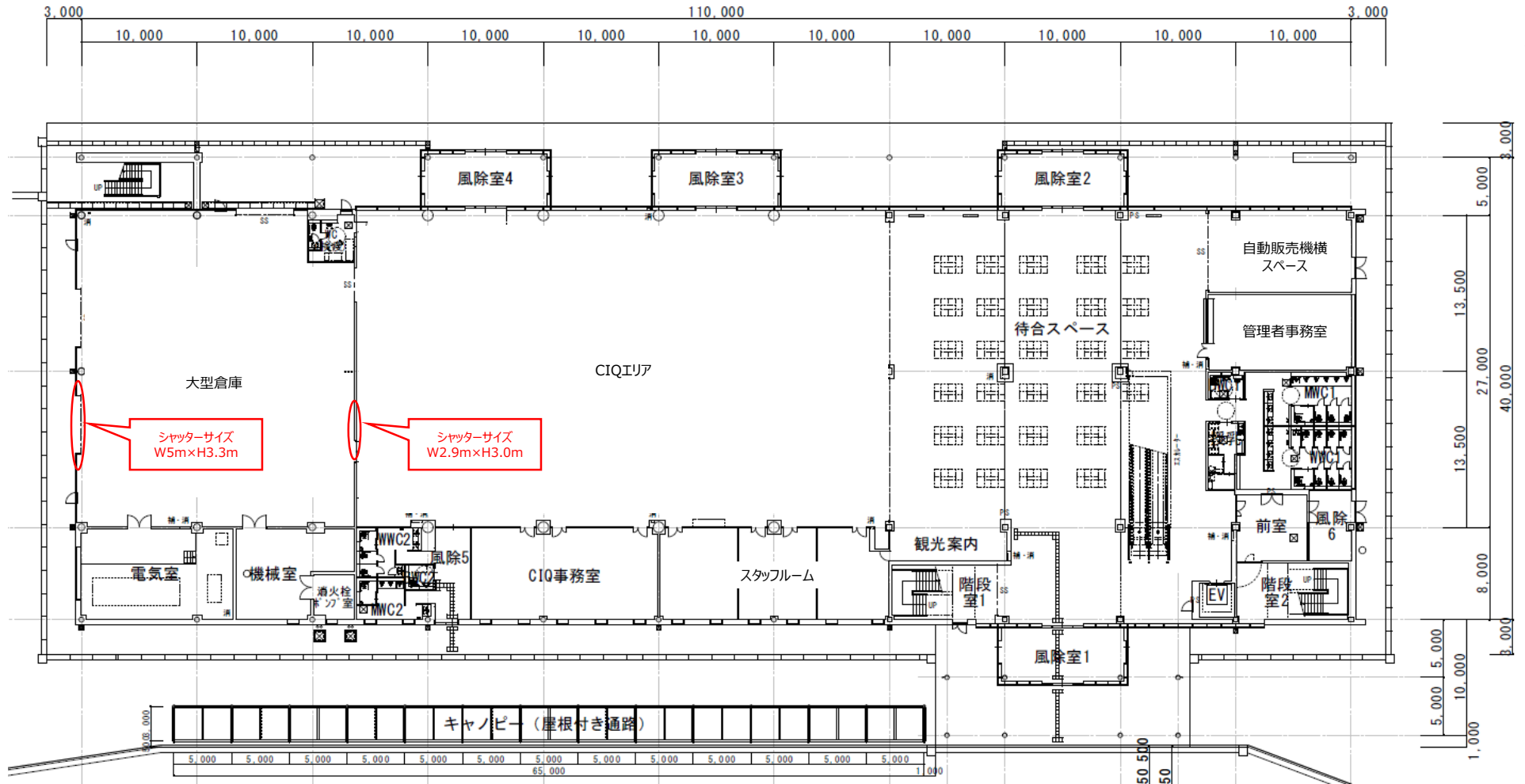
平面図（1階）
