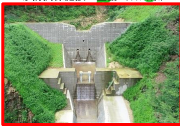
砂防関係施設の整備（石川県）
