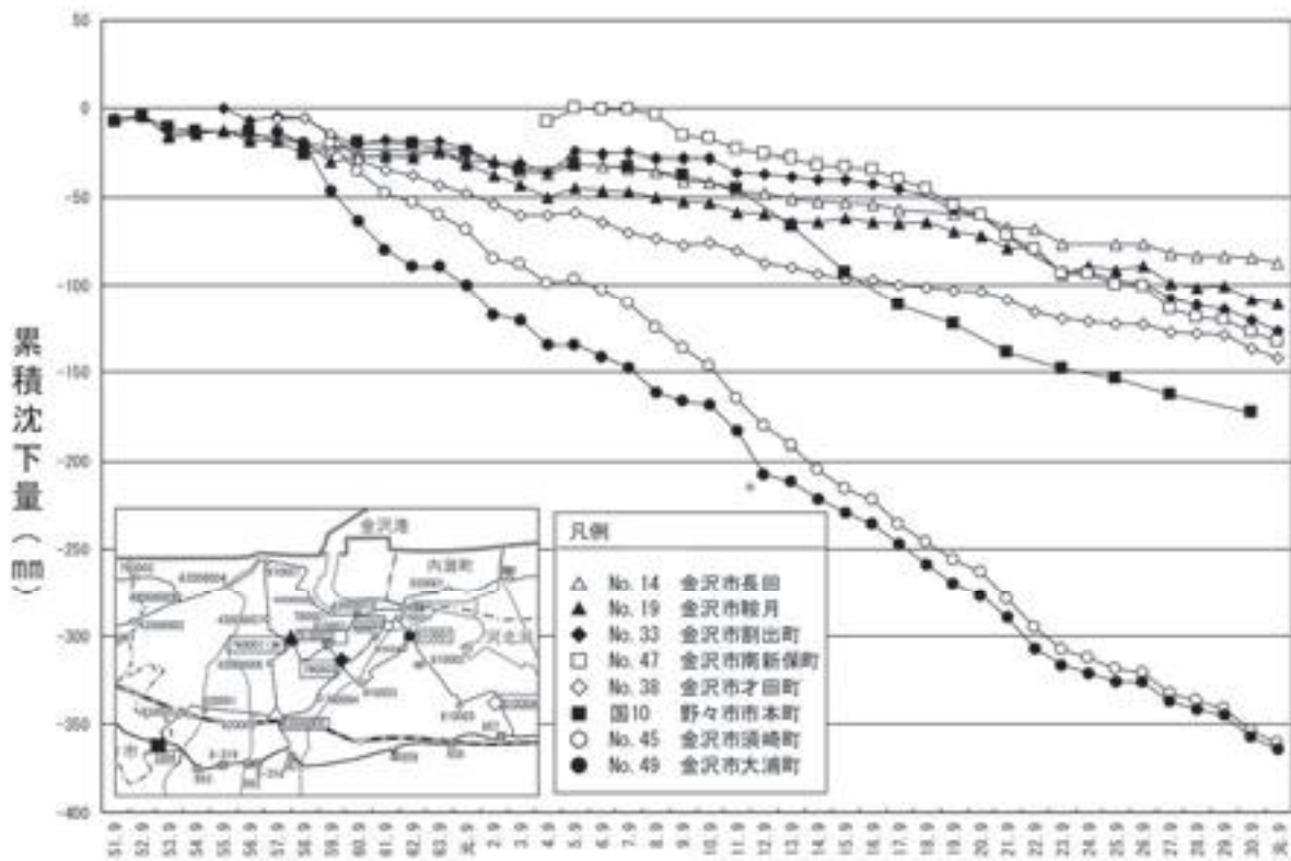
* 工事による影響 (H11) 図 2-2-1 (2) 主な水準点の累積地盤沈下量 (金沢市近郊)
