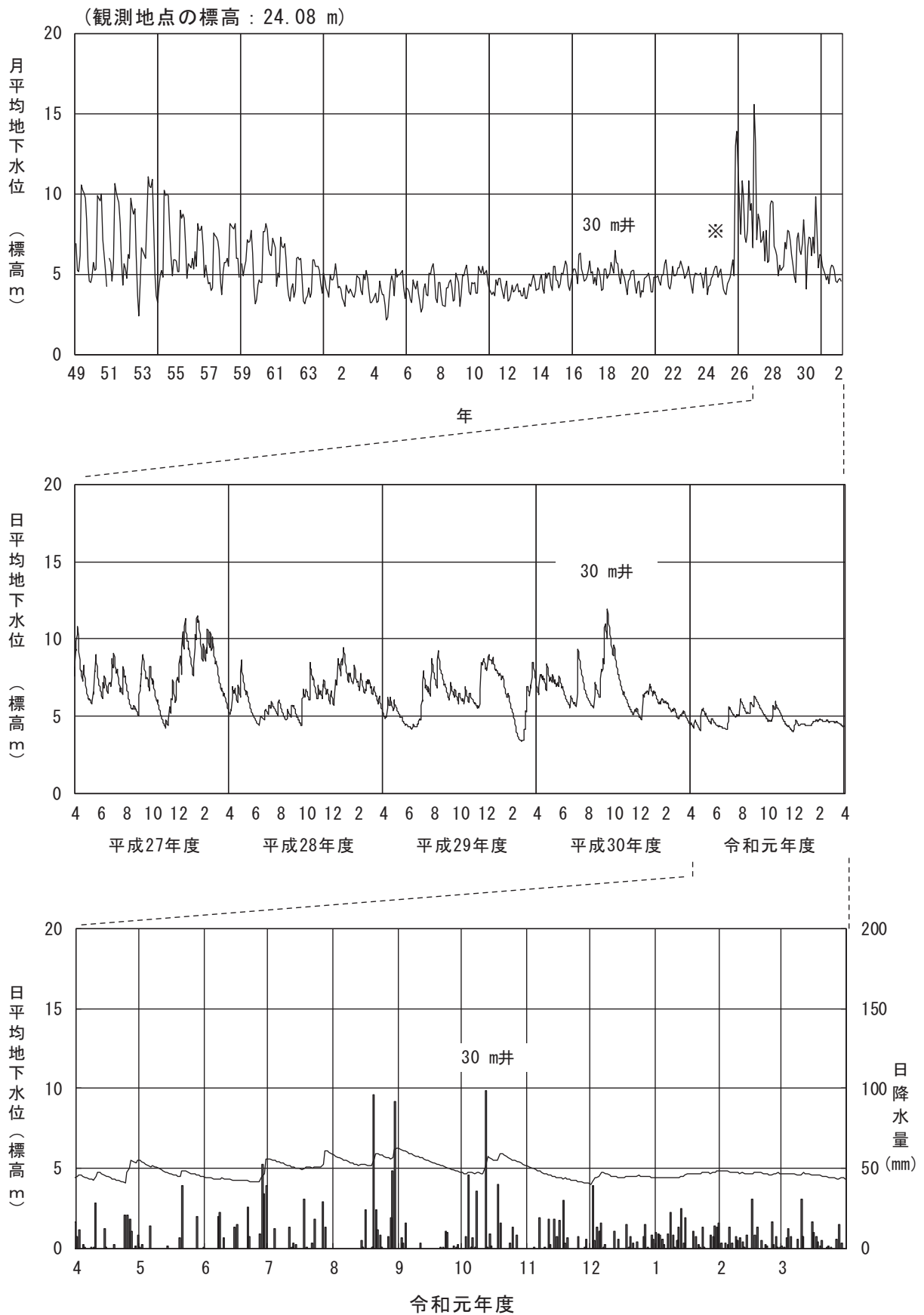
図 2-2-3 (17) 地下水位 (①白山市末広)
