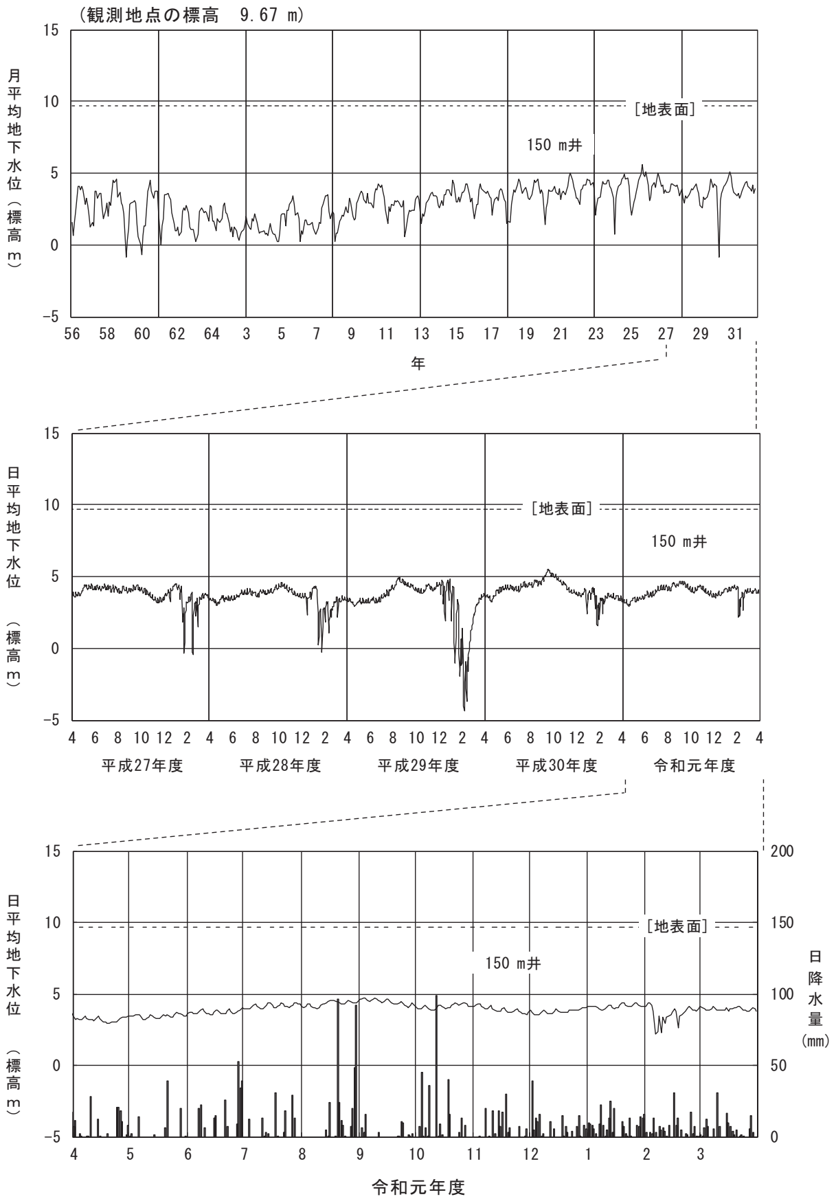
図 2-2-3(9) 地下水水位 (㊟金沢市新保本)
