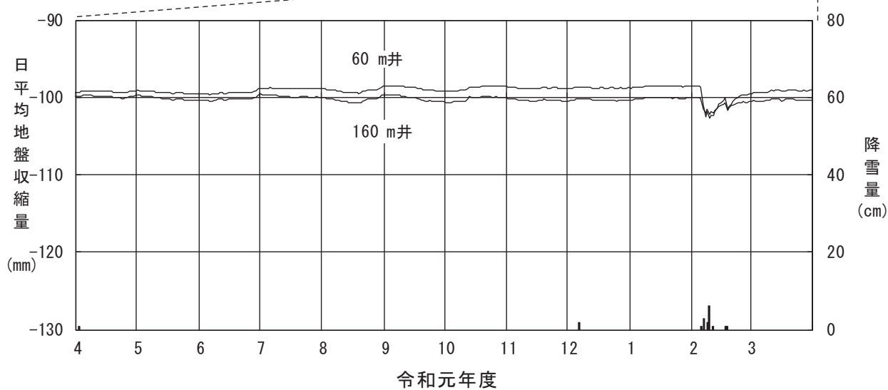
図 2-2-2 (3) 地盤収縮量 (③金沢市浅野本町)
