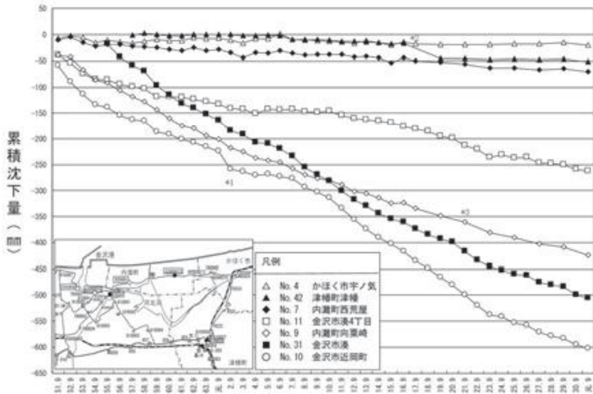
*1 工事による影響 (H2) *2 移設による欠測 (H17) *3 内灘町向栗崎は、平成 21 年 8 月までは 43008-011、平成 21 年 9 月以降は 92-0001 の水準点の値を累積 図 2-2-1 (1) 主な水準点の累積地盤沈下量 (津幡町横浜～金沢市湊町)
