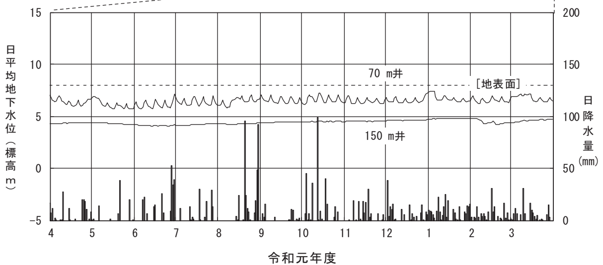
図2-2-3(21) 地下水位 (㊸能美市赤井)
