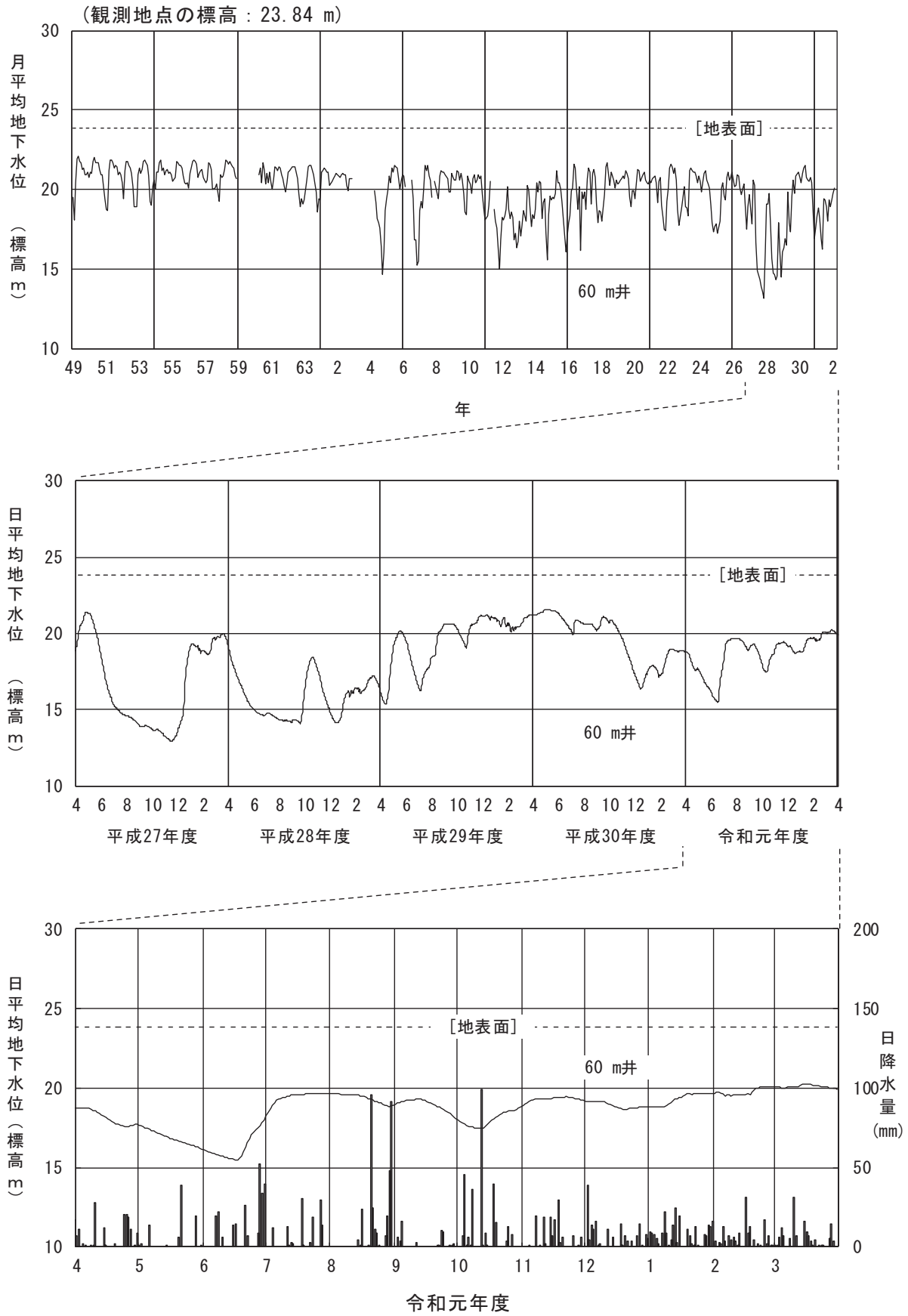
図 2-2-3 (22) 地下水位 (②能美市北市)
