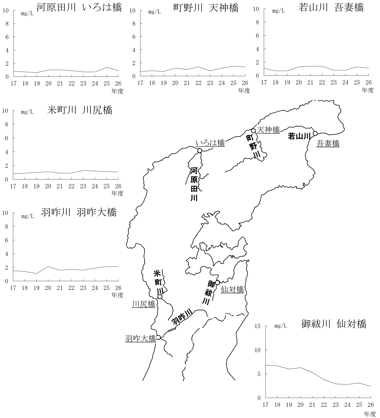
図一 9 能登地区河川のBOD経年変化 (年平均値)
