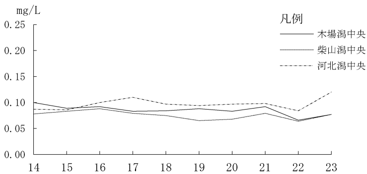
図-12 湖沼の全リン経年変化（年平均値）年度
