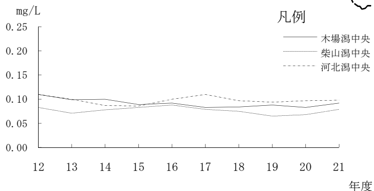
図-12 湖沼の全リン経年変化（年平均値）
