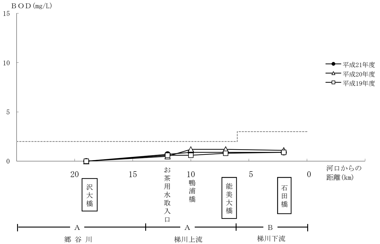
図-4 梯川水系のBOD変化（上流→下流）
