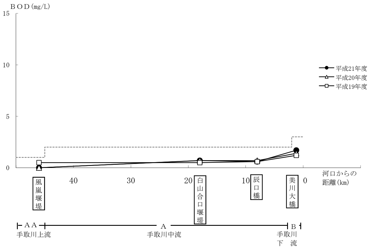
図-5 手取川水系のBOD変化（上流→下流）
