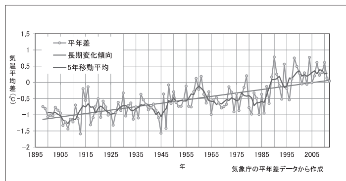
図1 日本の年平均気温の年差の経年変化（1900～2012年）
