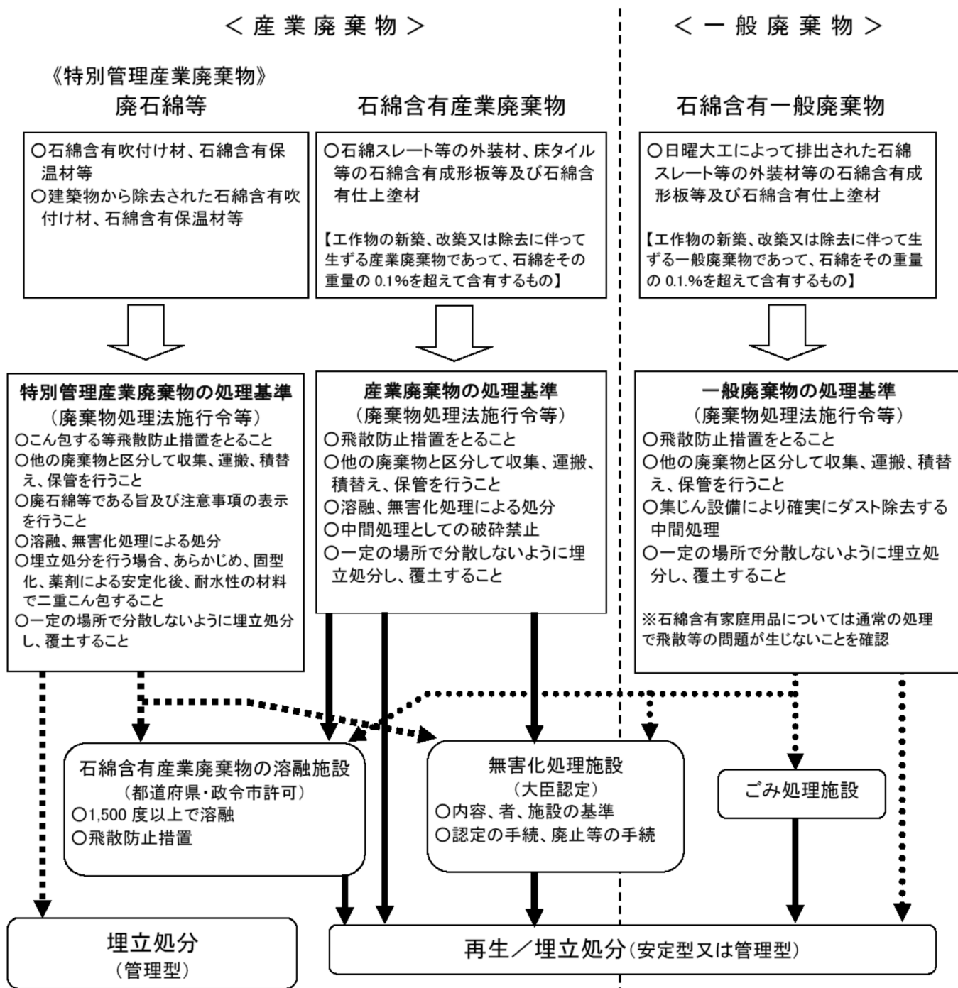
図－8 廃石綿等又は石綿含有廃棄物の処理フロー
