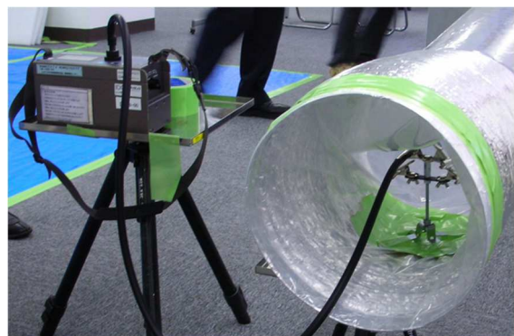
集じん・排気装置が正常に稼働していることの確認例 (デジタル粉じん計による確認)
