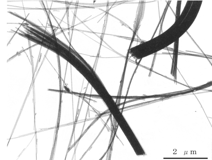
図-1 石綿（クリソタイル）の透過型電子顕微鏡写真
