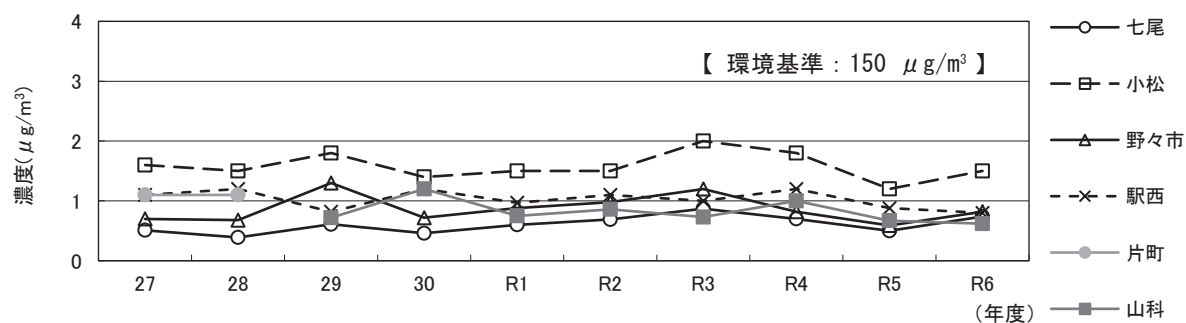
図 5-4 ジクロロメタンの経年変化
