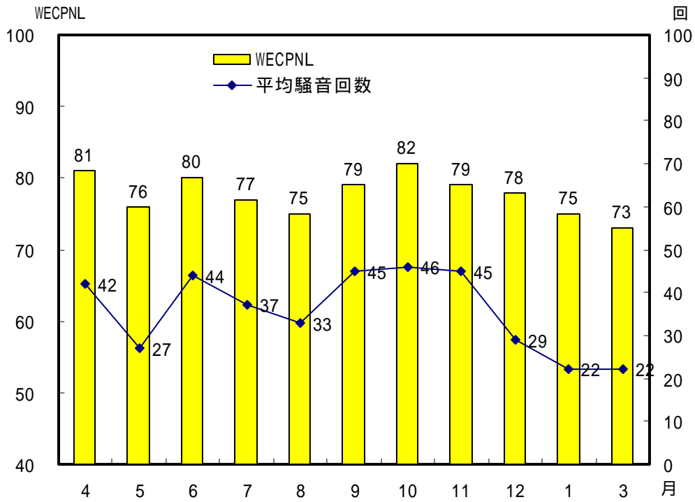
図 - 5 常時測定点における月別1日平均騒音発生回数とWECPNL (小松市小島町)
