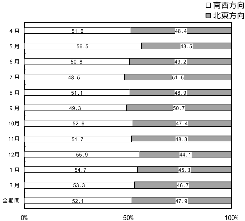
図 - 3 常時測定点における方向別騒音発生割合
