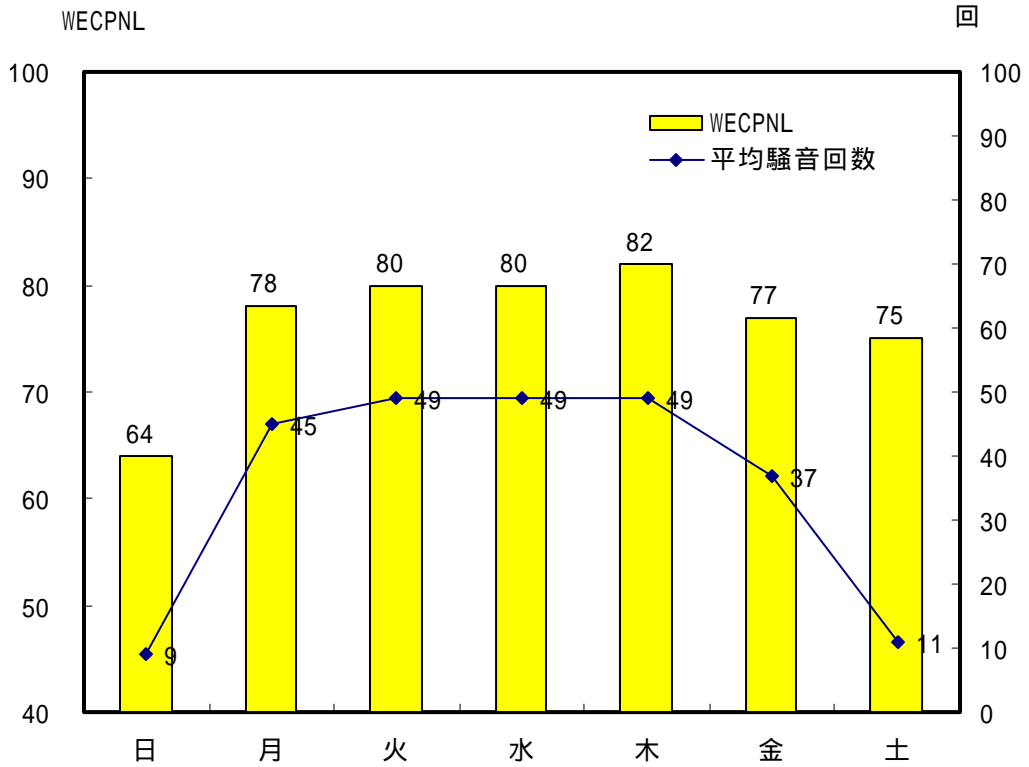
図 - 7 常時測定点における曜日別 1 日平均騒音発生回数と WECPNL ( 小松市小島町 )
