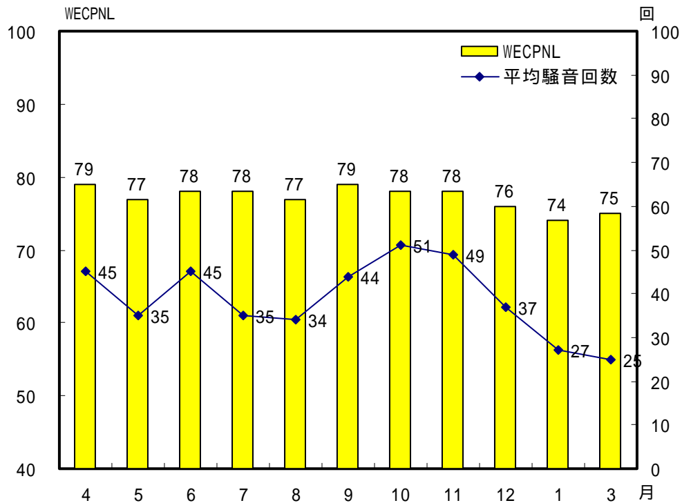
図 - 6 常時測定点における月別1日平均騒音発生回数とWECPNL (加賀市伊切町)
