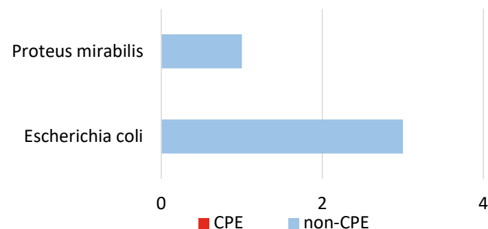
CREから検出されたカルバペネマーゼ遺伝子（菌種別）
