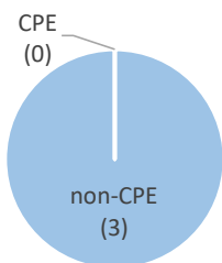
CREから検出されたカルバペネマーゼ遺伝子（全体）
