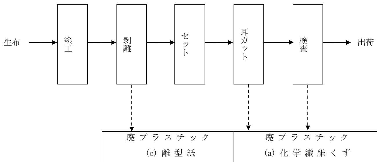
図 3. 複合薄膜加工フローシート (No. 2)
