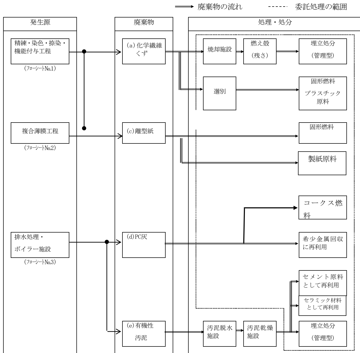
図 1. 廃棄物処理フローシート (現行)
