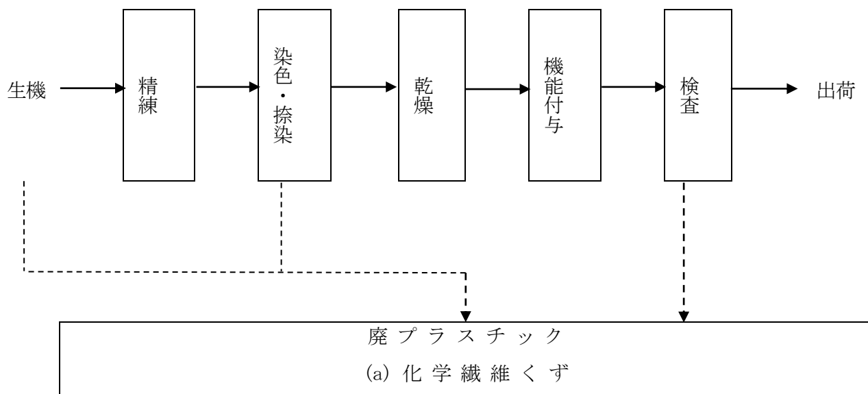
図 2. 染色・捺染・機能付与加工工程フローシート (No. 1)
