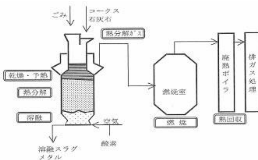
図1 シャフト式ガス化溶融炉システムのフロー例
