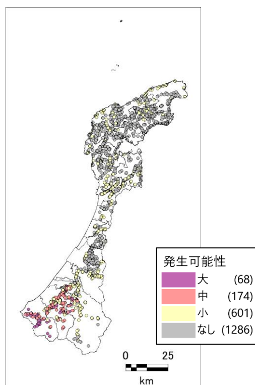
図 2.3-54 土石流
