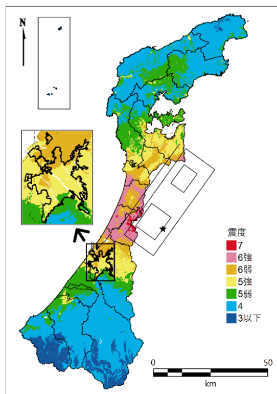
図 2.1-7 地表震度分布 邑知湊断層帯
