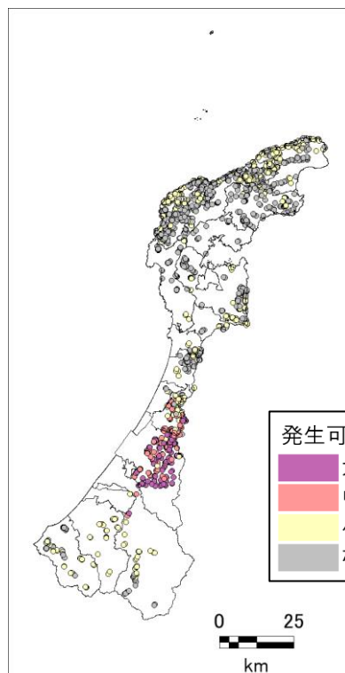
図 2.3-35 地すべり
