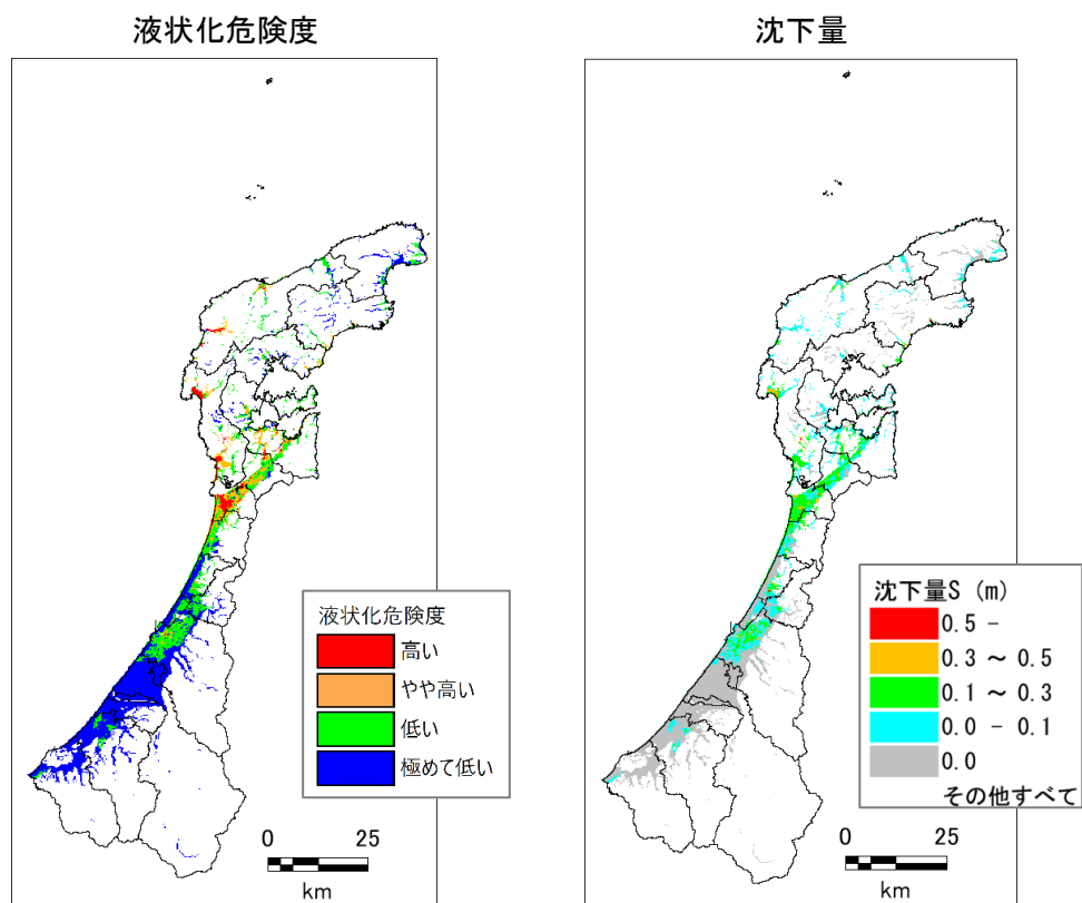
図 2.2-16 門前断層帯(西上部に震源)の液化化分布
