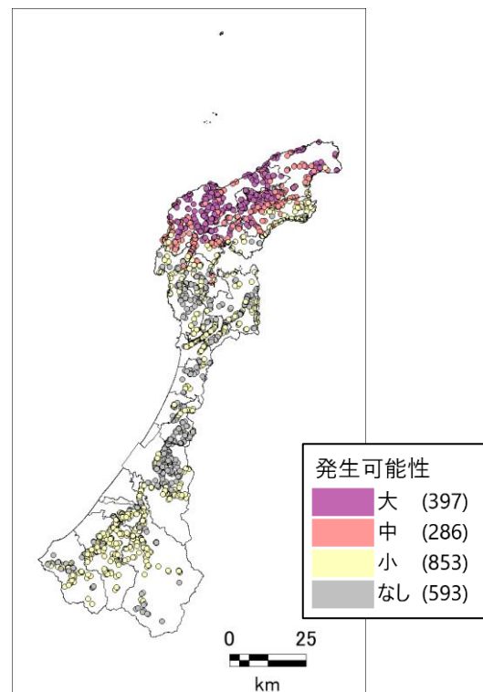
図 2.3-87 土石流
