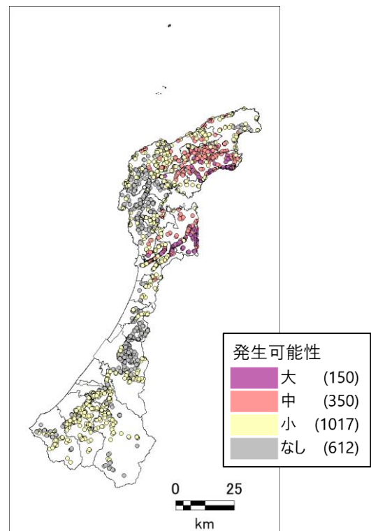
図 2.3-105 土石流
