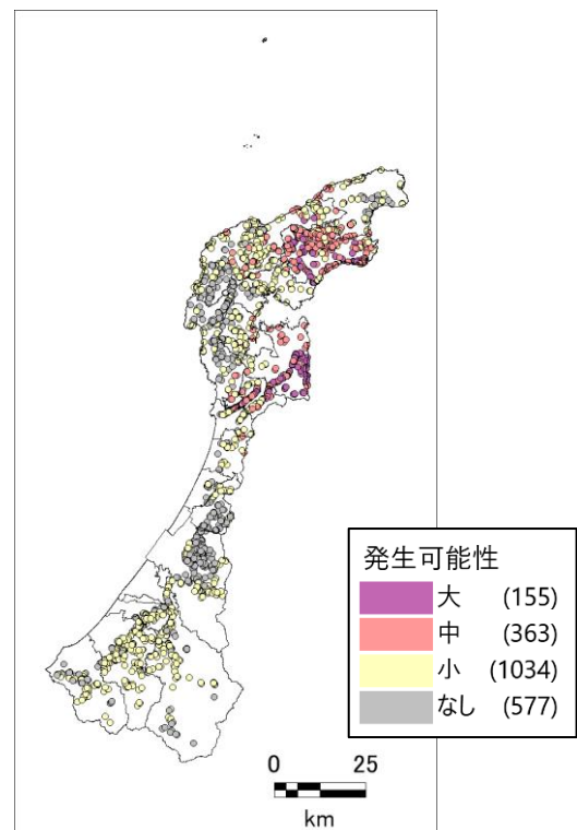
図 2.3-99 土石流
