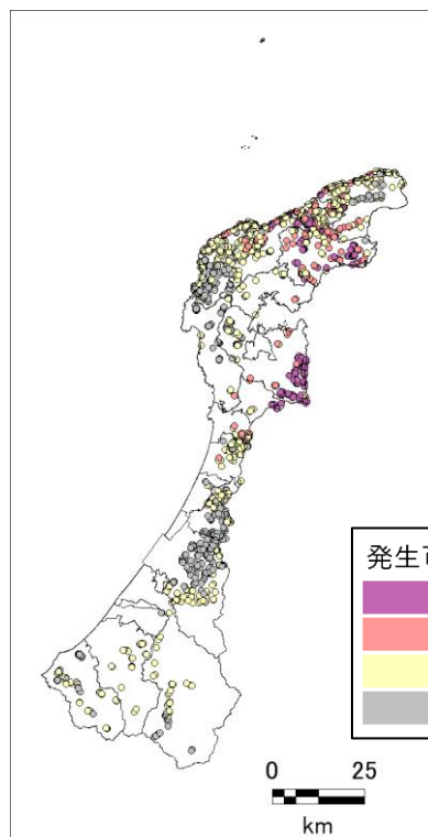
図 2.3-98 地すべり
