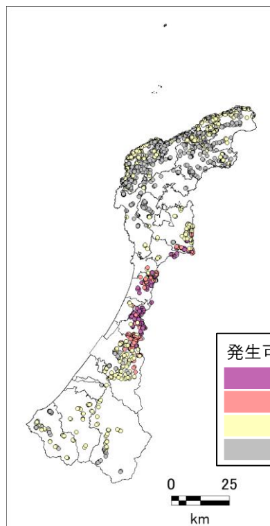
図 2.3-41 地すべり
