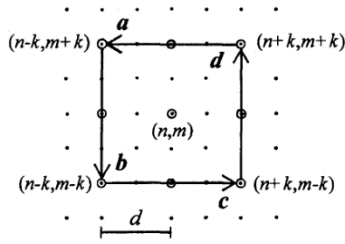
図-5 斜度の計算に用いた節点配置 ( n, m ) は節点の座標番号。黒点は節点の位置。白点は近傍節点。 d は近傍節点の距離。 k はそのメッシュ数 (この図の場合は 2)。 a, b, c, d は近傍節点同士を結ぶベクトル。
