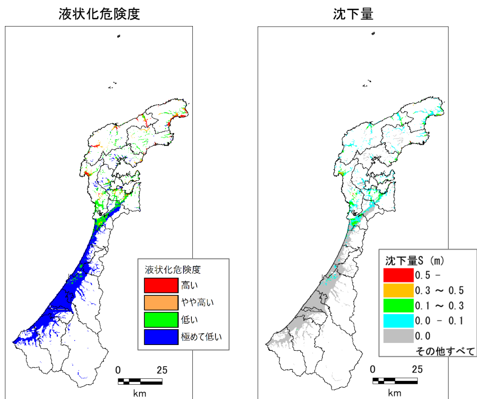
図 2.2-17 能登半島北岸断層帯(南下部に震源)の液化化分布
