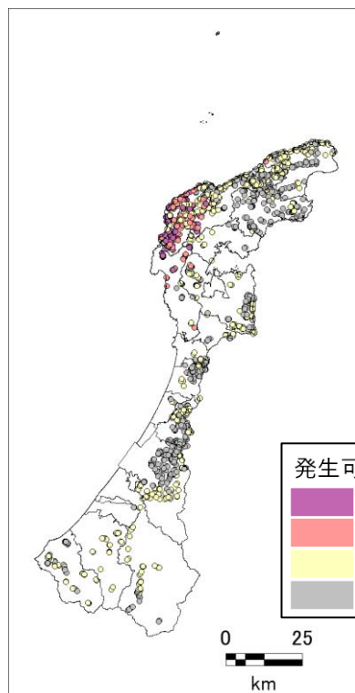
図 2.3-71 地すべり
