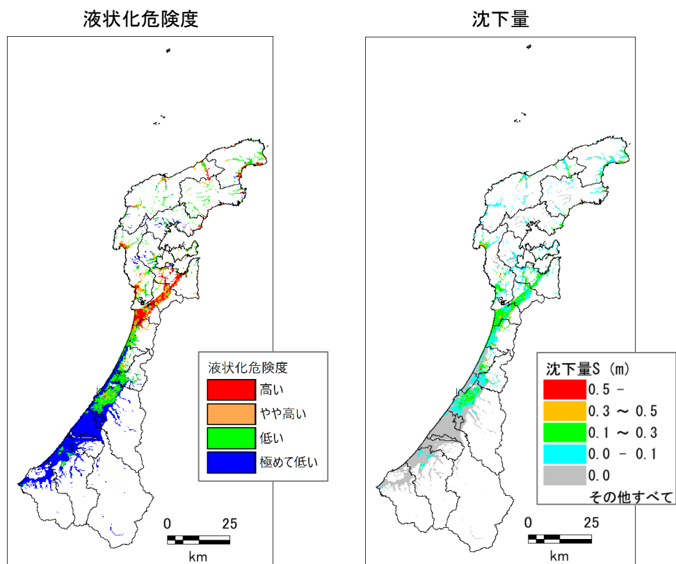
図 2.2-26 七尾湾東方断層帯(南上部に震源)の液化化分布
