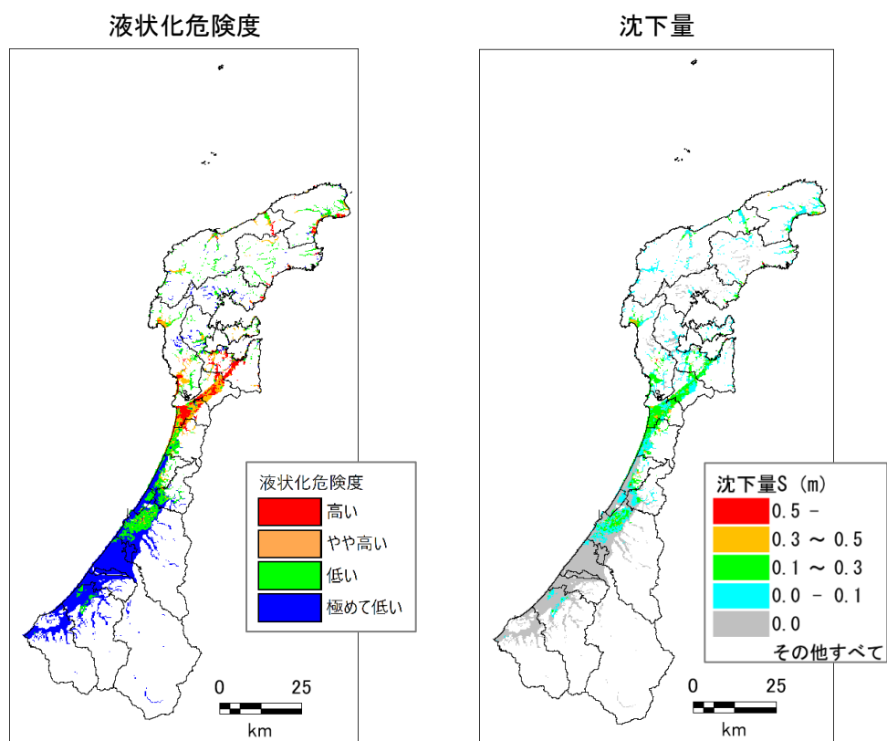
図 2.2-27 七尾湾東方断層帯(北下部に震源)の液化化分布
