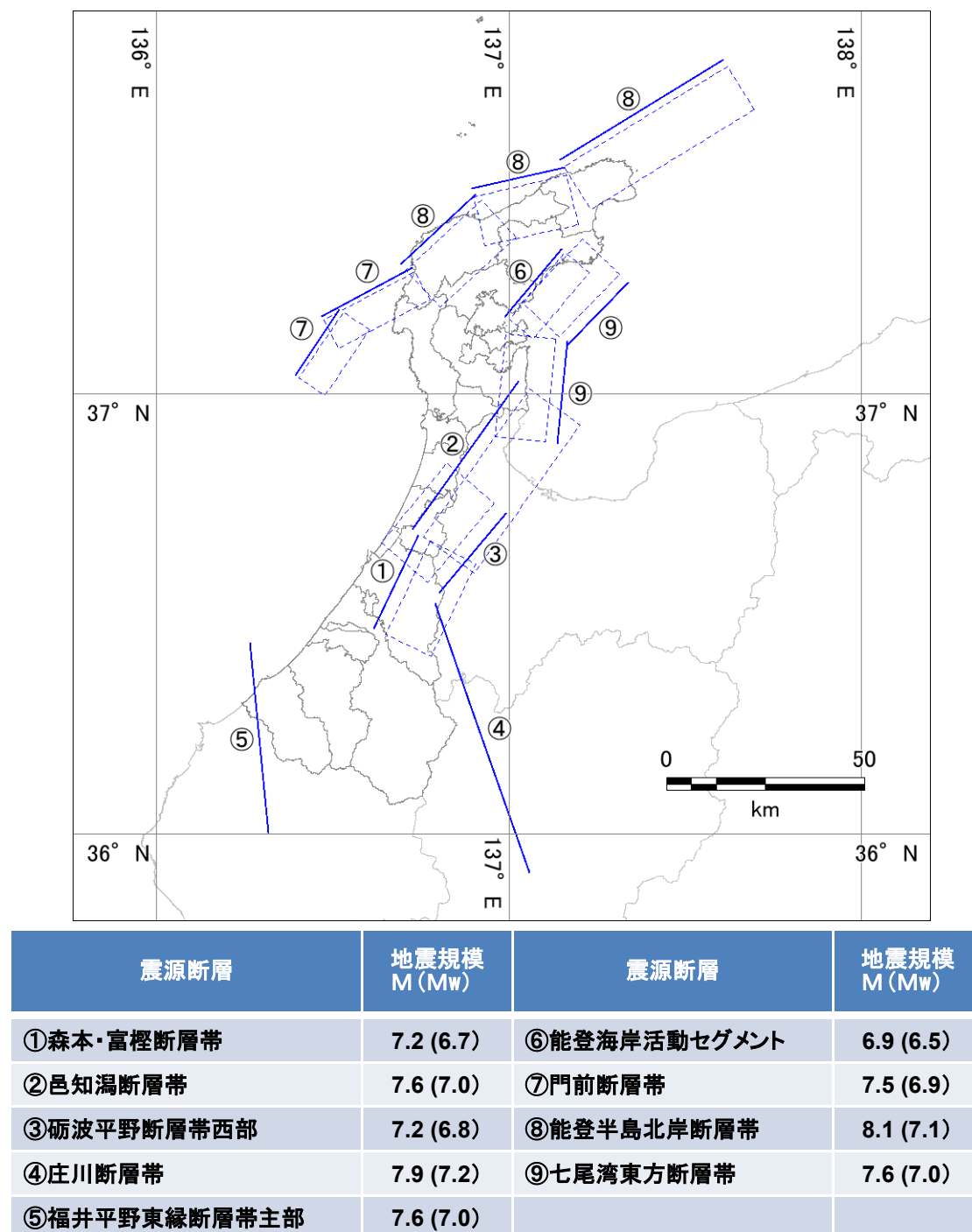
図 2.1-3 想定地震の一覧
