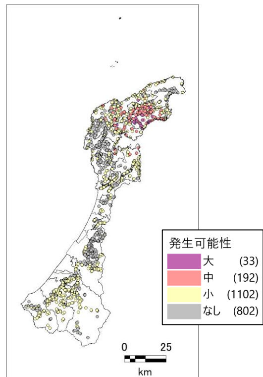
図 2.3-60 土石流
