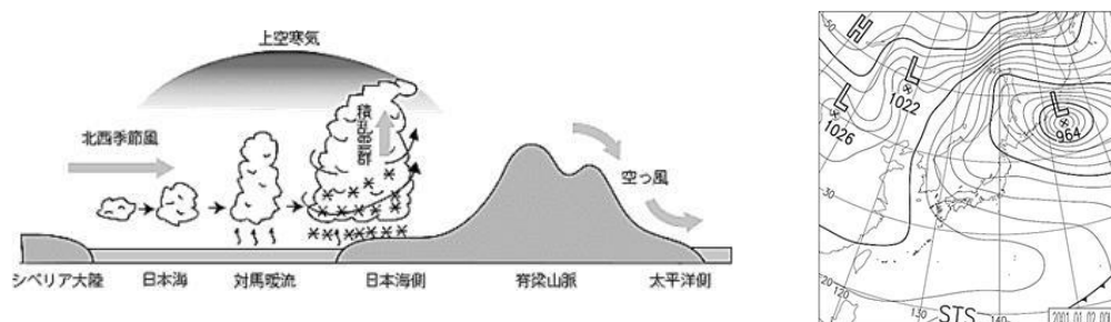
図2 里雪型の概念図（右）と気圧配置（左）（参考〔2〕）
