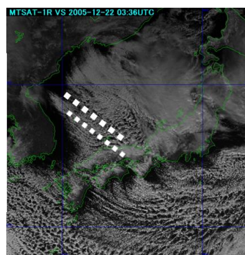
図4 気象衛星画像（可視）
