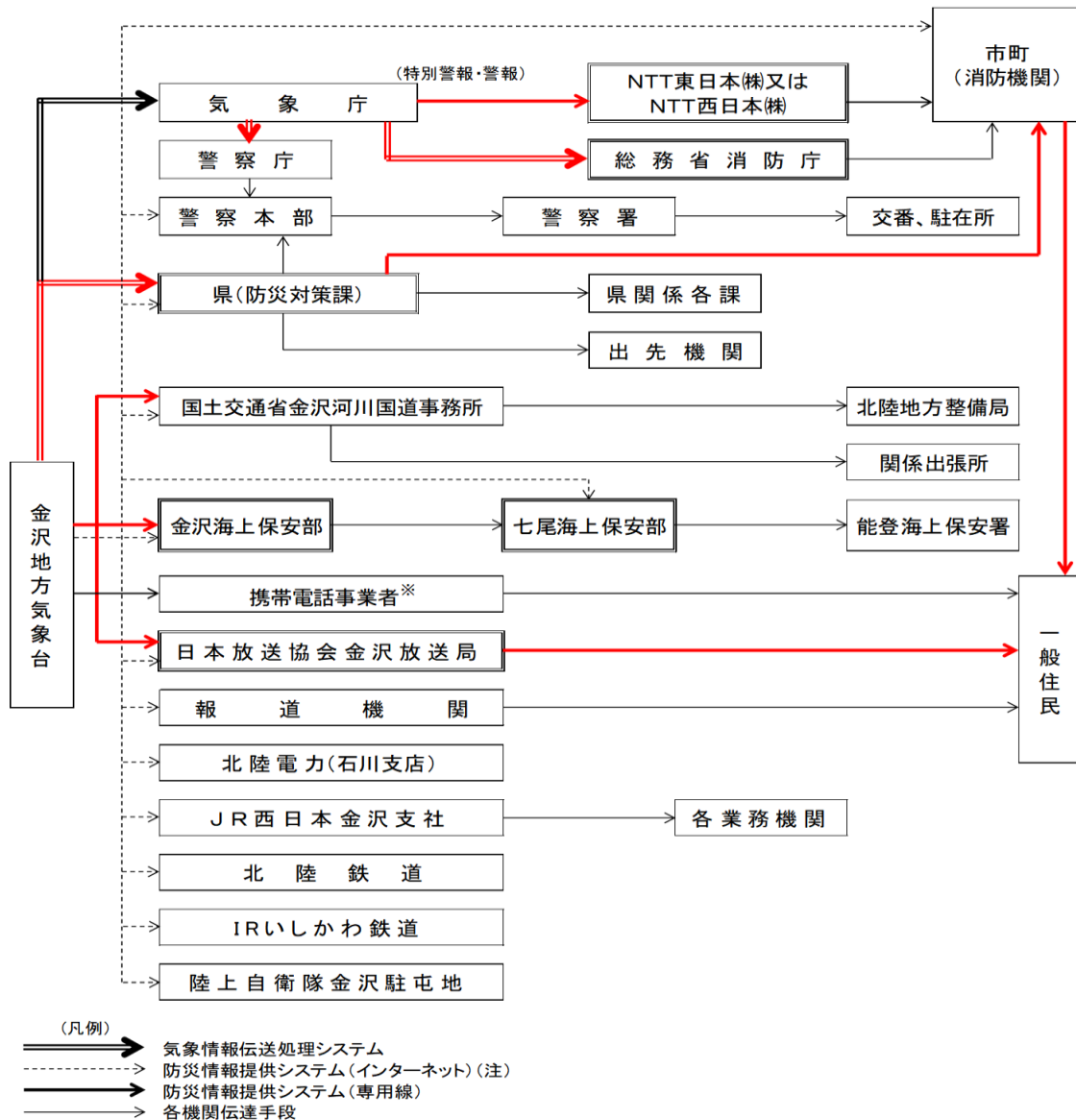
別図1 金沢、七尾海上保安部を中心とする気象警報等伝達系統図
