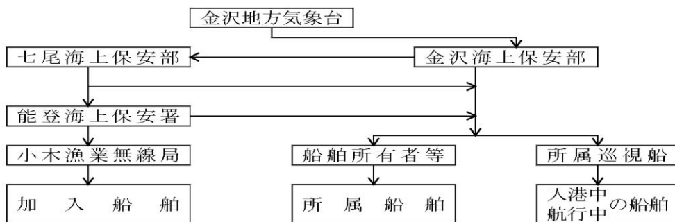
別図2 金沢、七尾海上保安部を中心とする気象警報等伝達系統図
