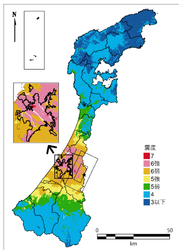
④ 庄川断層帯
