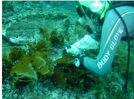
藻場の調査
