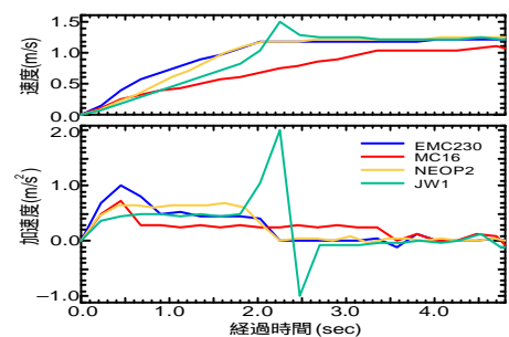
電動車いす駆動特性計測データ
